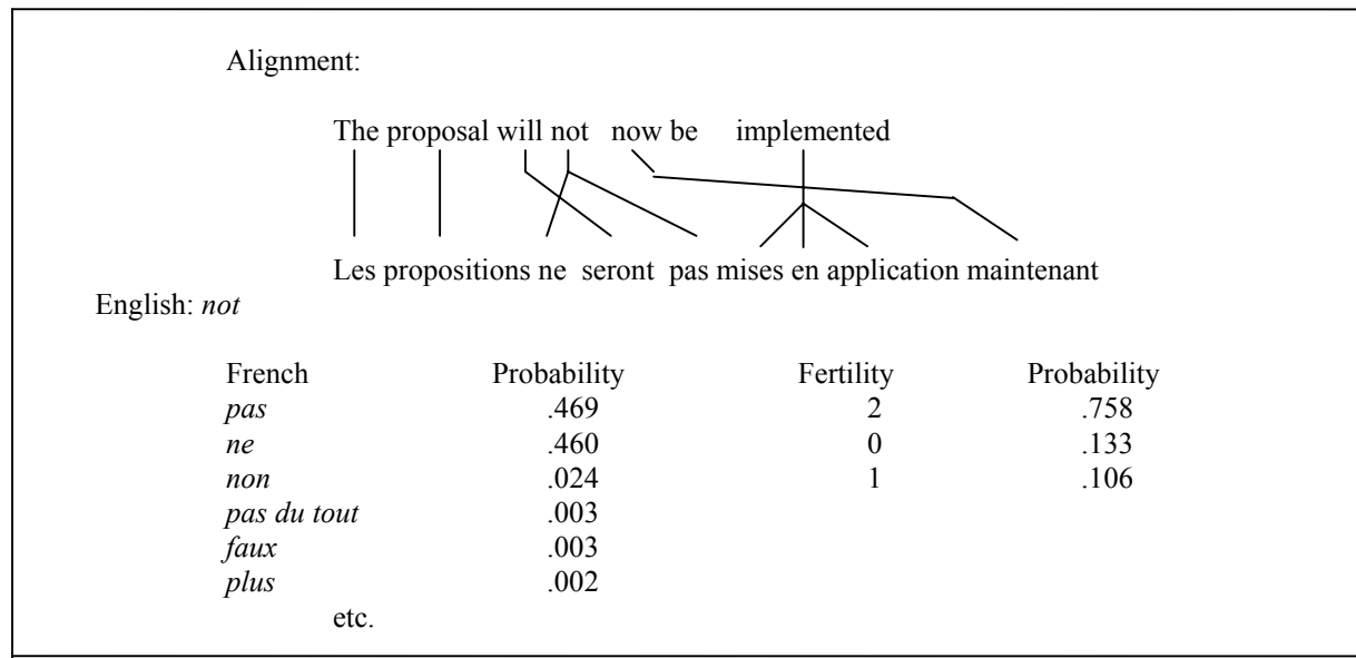
Fig. 4 Stochastic MT ( Candide , IBM)
